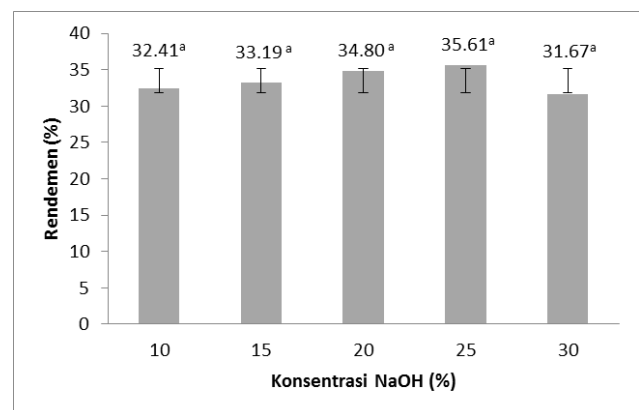
Gambar 2. Grafik Rendemen Ekstraksi Selulosa Batang Jagung
