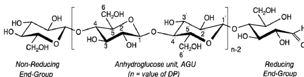
Gambar 1. Struktur Molekul Selulosa (Coffey et al , 1995)
