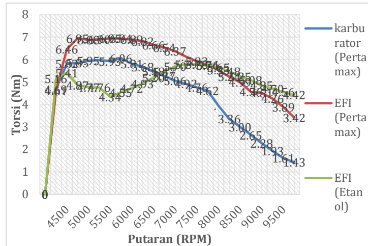
Gambar 2. Hasil pengujian torsi (Nm) pada sistem konvensional, EFI dan EFI dengan bahan bakar etanol.
