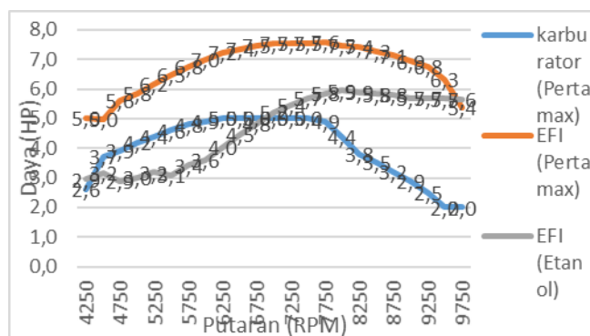
Gambar 3. Hasil pengujian daya pada sistem konvensional, EFI dan EFI dengan bahan bakar etanol.
