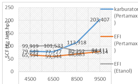
Gambar 4. Hasil pengujian konsumsi bahan bakar pada sistem konvensional, EFI dan EFI dengan bahan bakar etanol.
