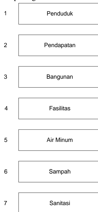
Gambar 2. Perancangan entity
