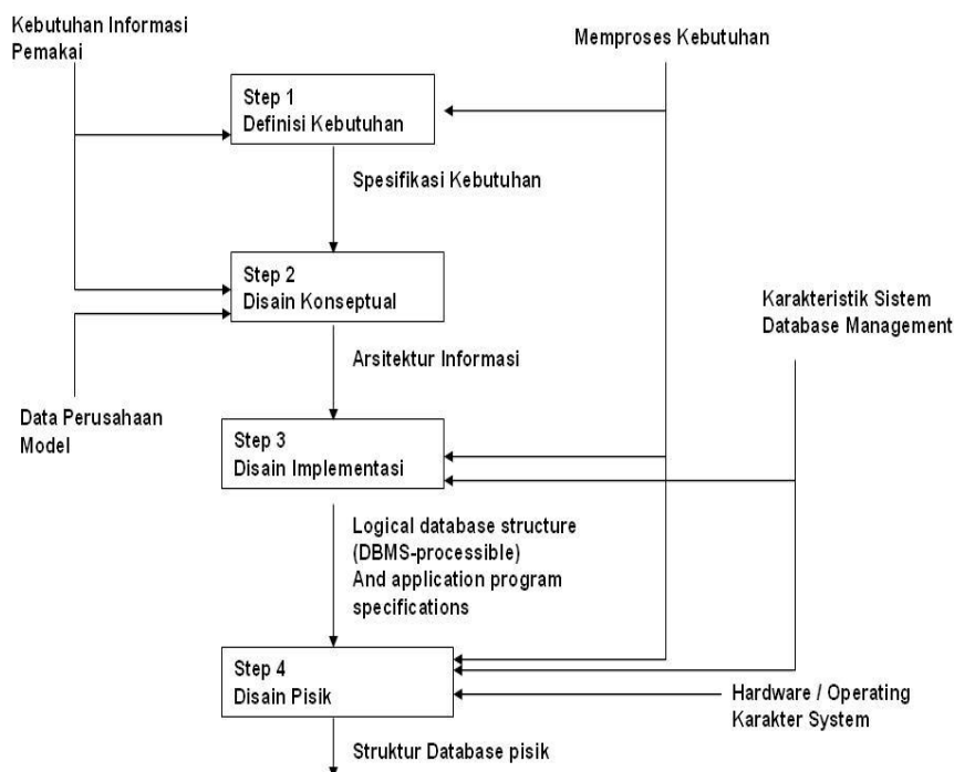
Gambar 1. Perancangan Database
