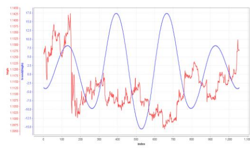
Gambar 6 kernel Epachnenikof
