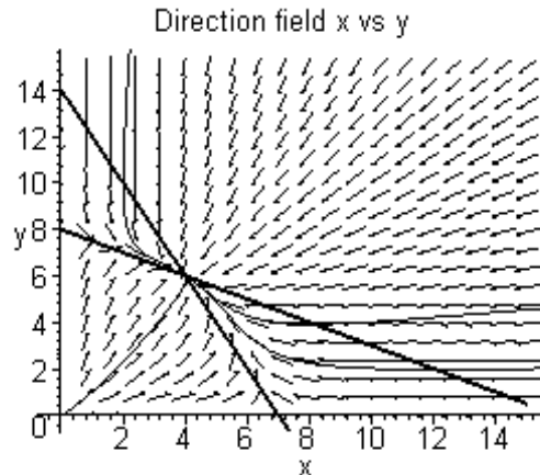
Gambar 4. Kasus dimana x(t) dan y(t) akan hidup berdampingan
