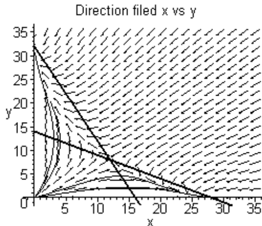
Gambar 3. Kasus dimana salah satu dari x(t) atau y(t) akan punah
