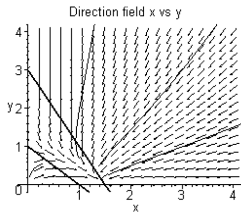
Gambar 2. Kasus dimana y(t) akan punah
