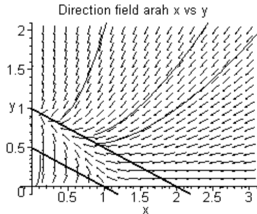
Gambar 1. Kasus dimana x(t) akan punah
